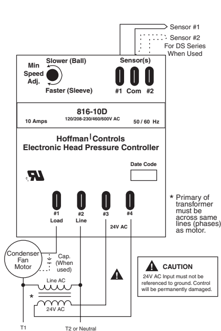
Figure 1 Wiring for 816-10D and 816-10DDS
